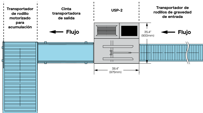
Plano típico de transportador para alimentar y retirar bandejas
